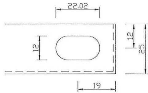
取付部詳細
